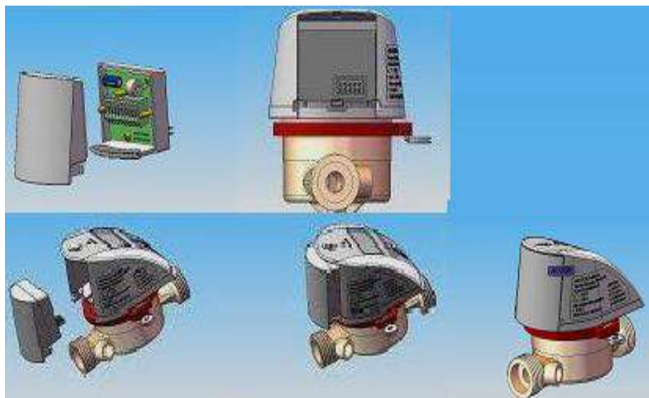
Рисунок 3. Размещение интерфейса.
