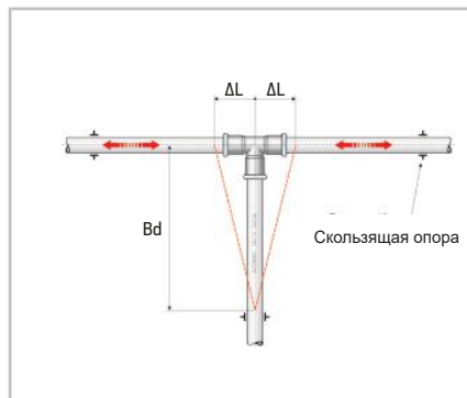
Рис. 47. Т-образный компенсатор.
