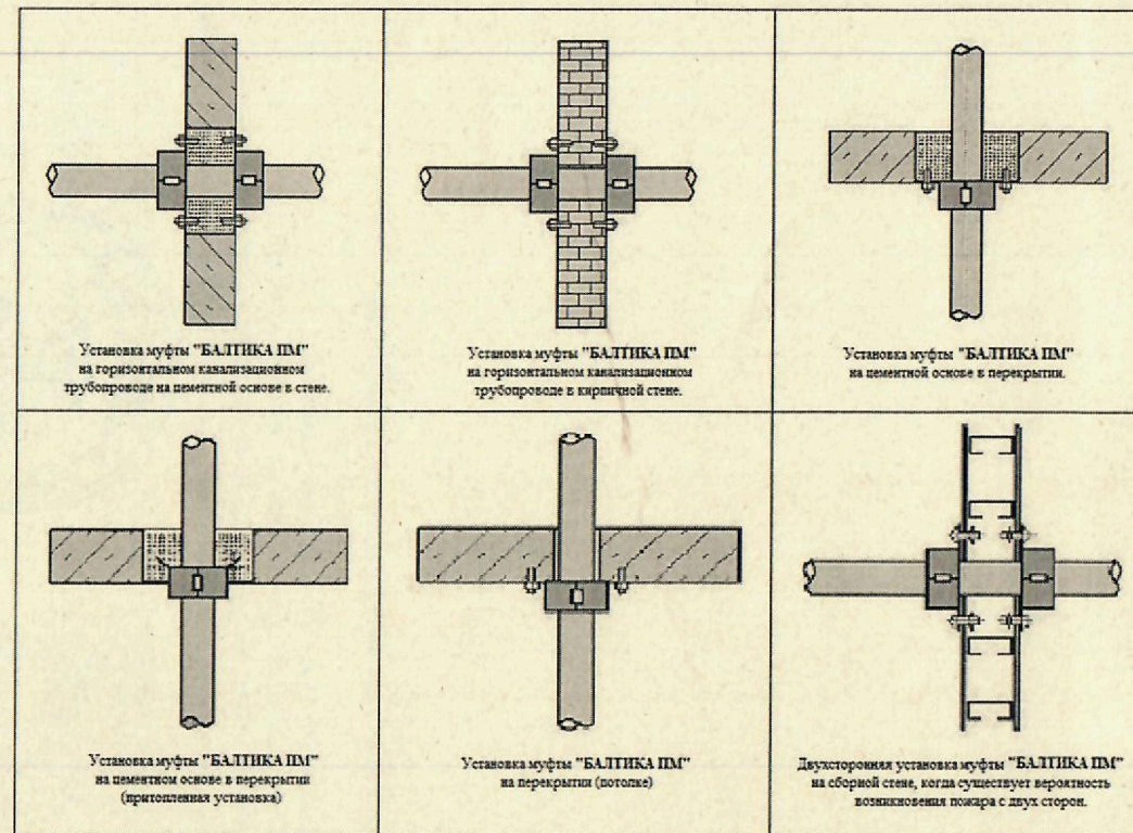
Схема установки 1
